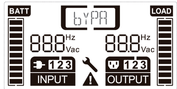
Fig. 15. Pantalla del modo de trabajo de modo Bypass.
