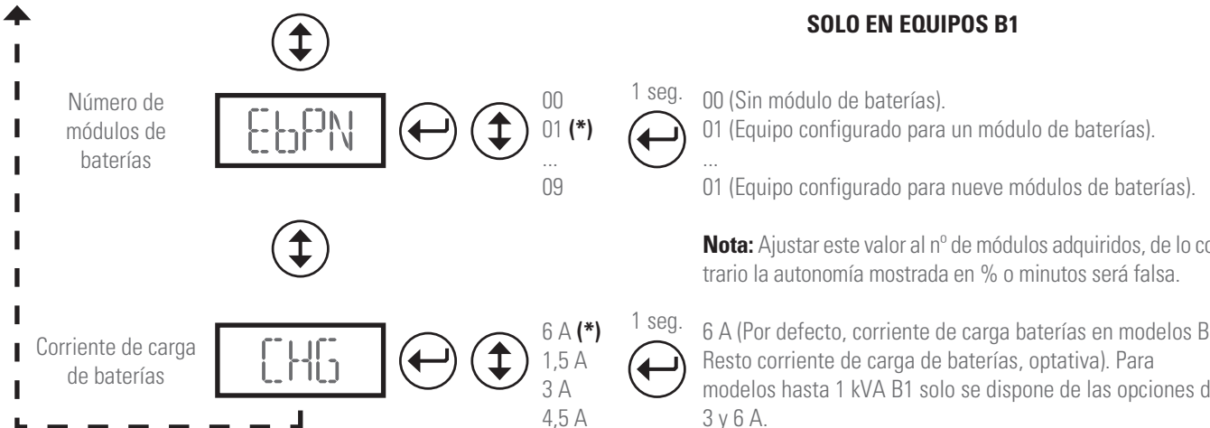
Fig. 20. Mapa de pantallas de ajuste.
