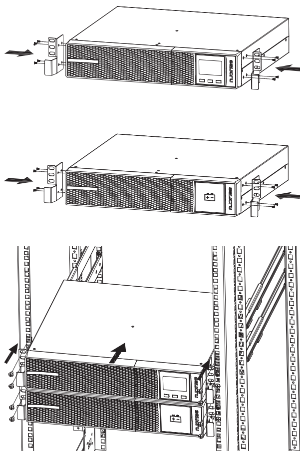
Fig. 5. Montaje tipo rack en armario 19", con extensión autonomía (módulo de baterías).
