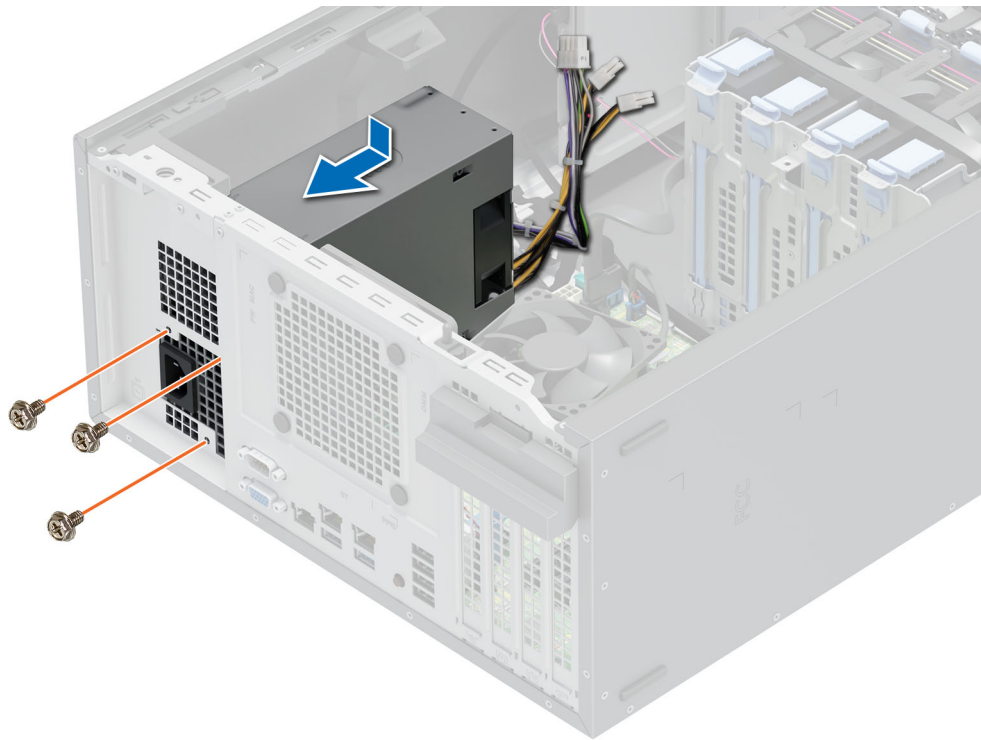
Ilustración 49. Instalación de la PSU D12
