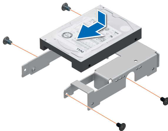
Ilustración 17. Instalación de una unidad de 2,5 pulgadas en el adaptador de unidad de 3,5 pulgadas
