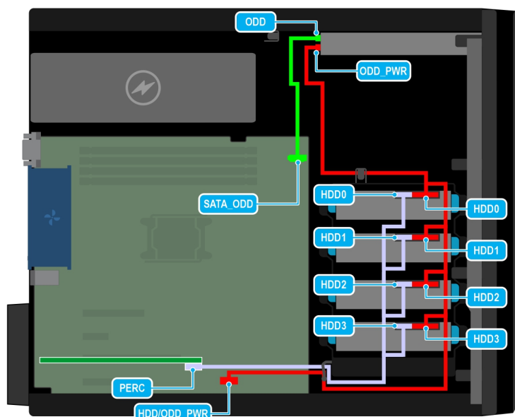
Ilustración 21. Colocación de los cables: disco SAS cableado de 4 x 3,5 pulgadas con tarjeta controladora de almacenamiento
