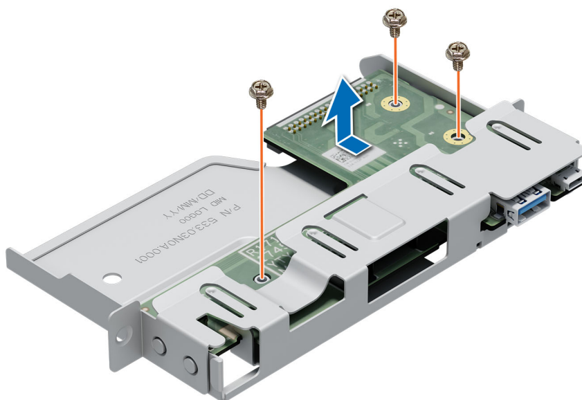
Ilustración 60. Extracción del panel de control
