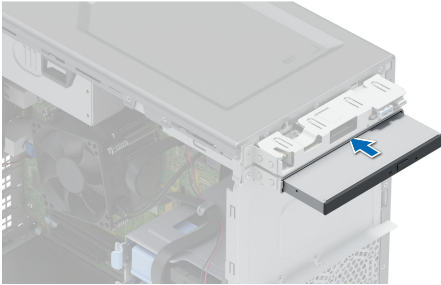
Ilustración 27. Instalación de las unidades ópticas
