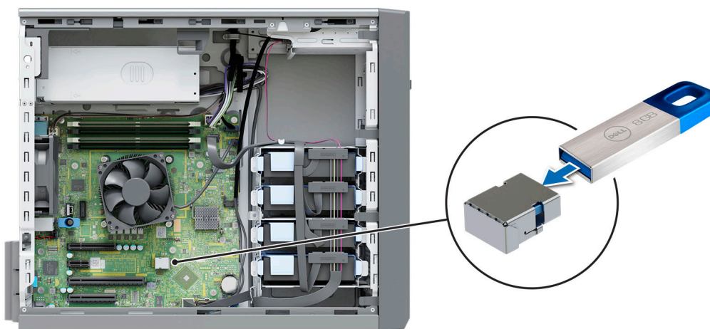
Ilustración 35. Instalación de la llave de memoria USB interna
