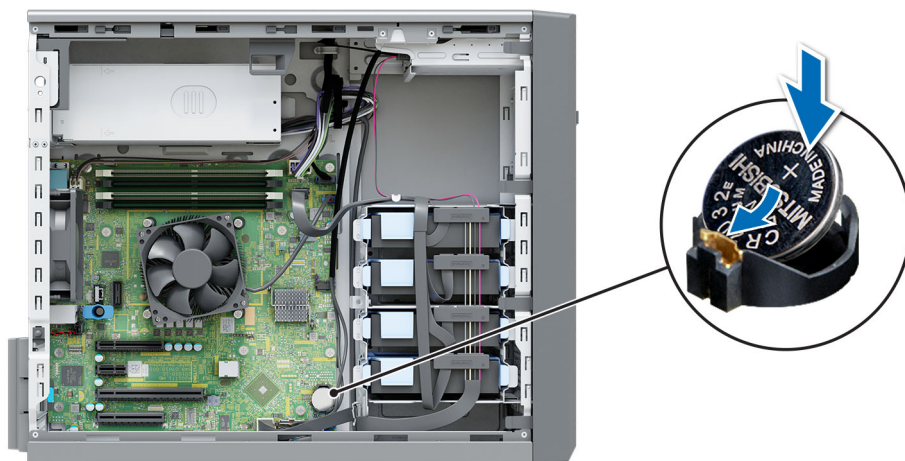
Ilustración 51. Instalación de la batería del sistema
