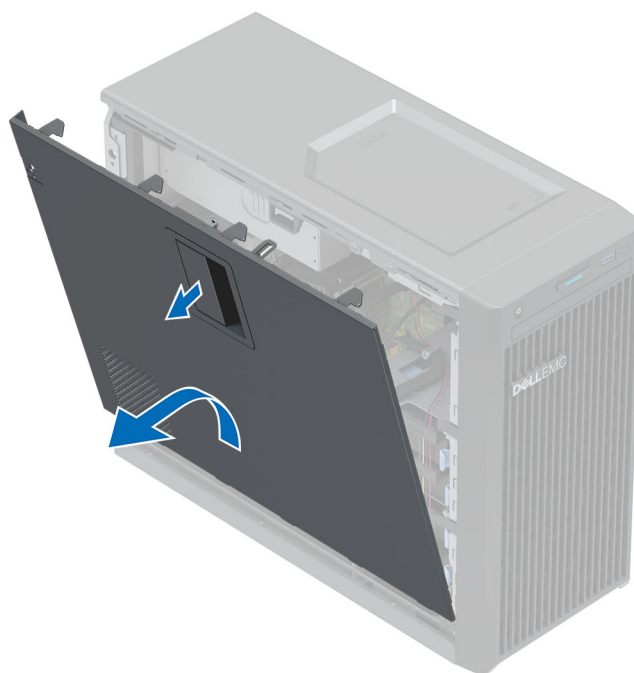
Ilustración 8. Extracción de la cubierta del sistema
