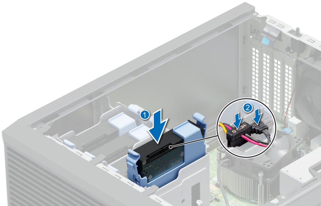
Ilustración 13. Instalación de un portaunidades en la bahía de unidad
