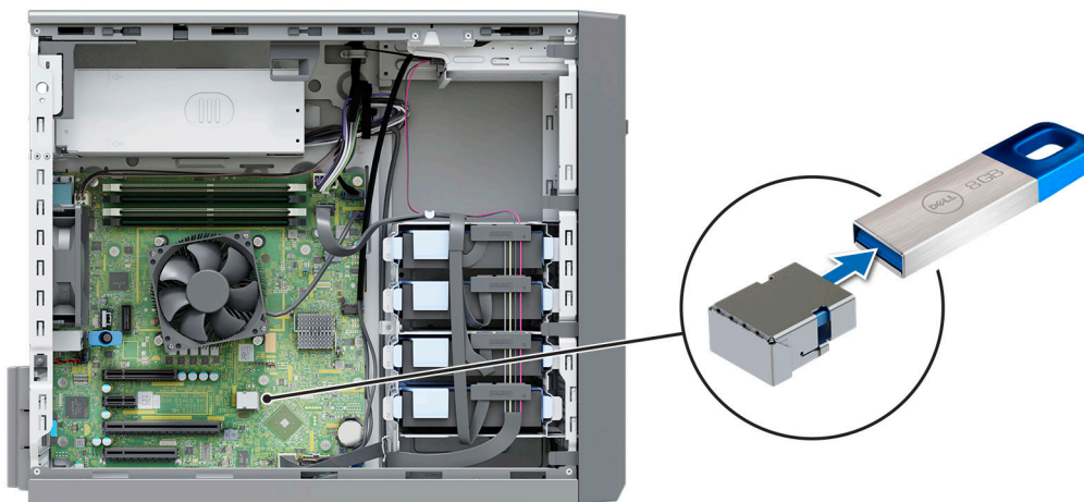
Ilustración 34. Extracción de la llave de memoria USB interna
