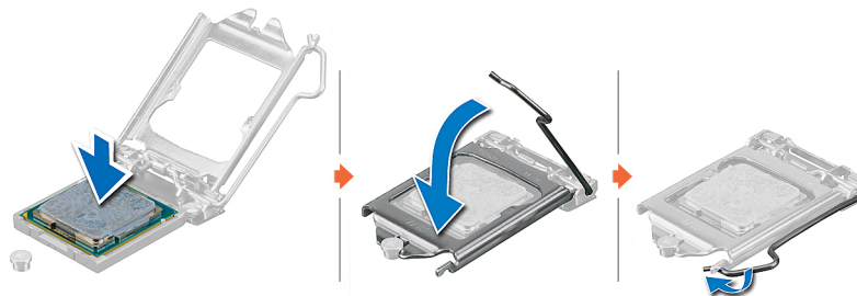
Ilustración 45. Instalación del procesador
