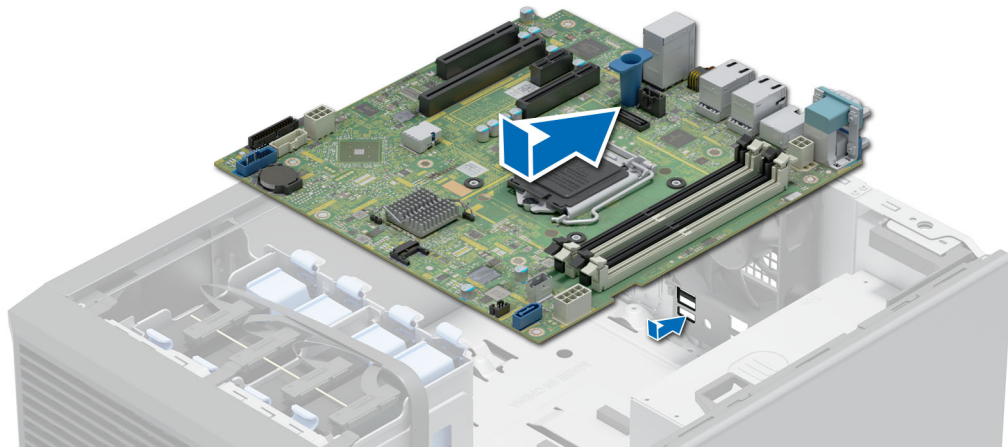
Ilustración 56. Instalación de la tarjeta madre
