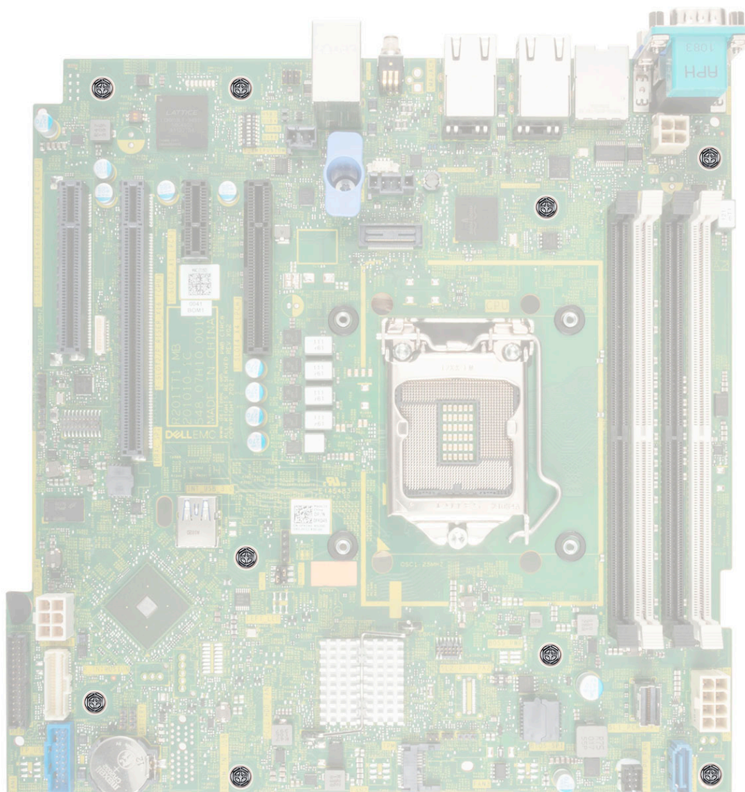
Ilustración 54. Ubicación del tornillo de la tarjeta madre
