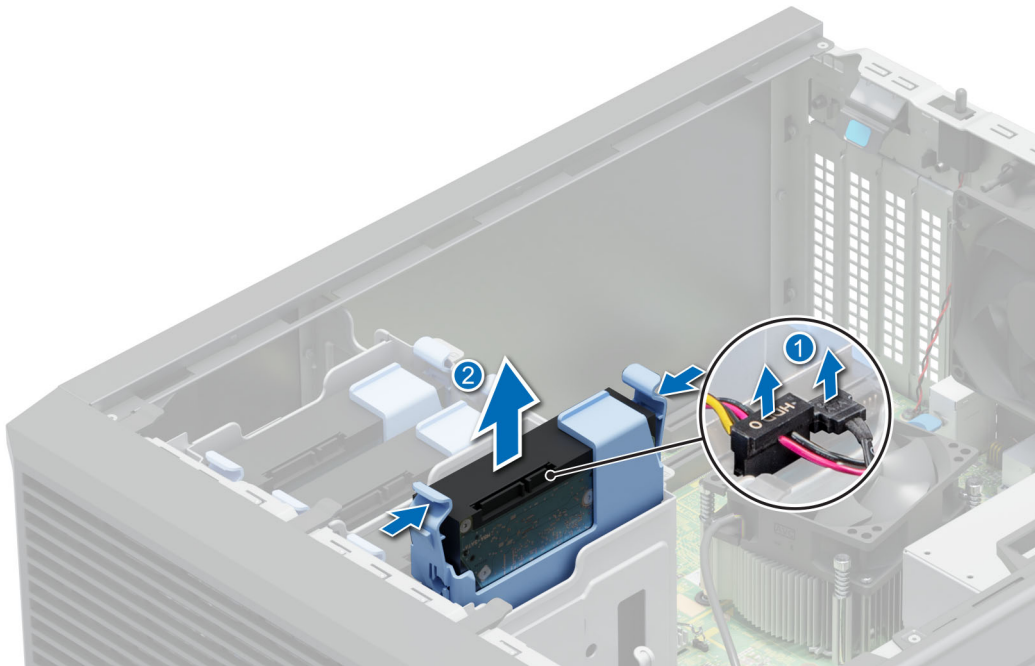
Ilustración 12. Extraiga el portaunidades de la bahía de unidad.
