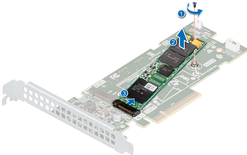
Ilustración 41. Extracción del módulo de SSD M.2
