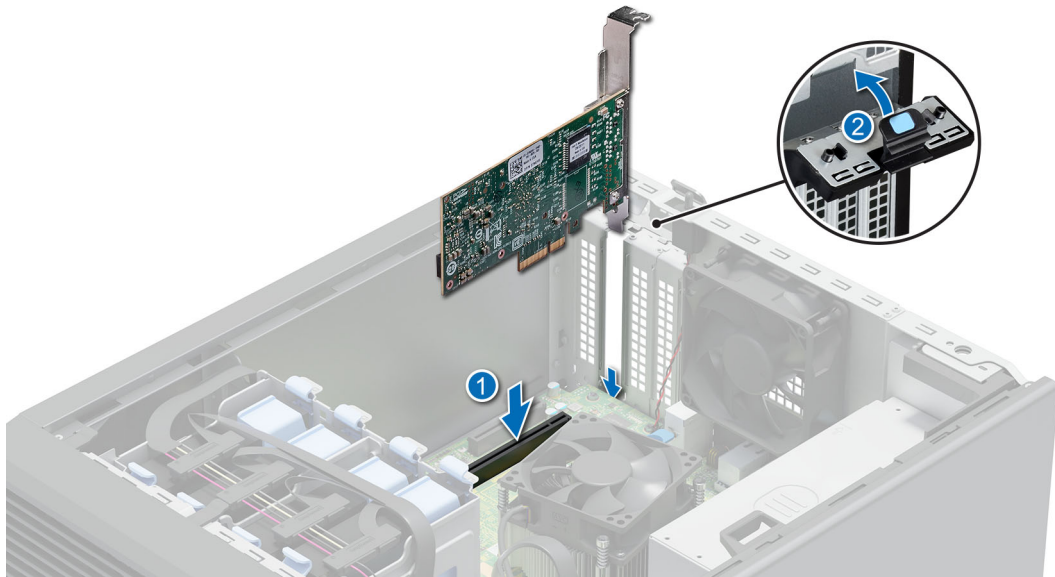
Ilustración 40. Instalación de la tarjeta de expansión PCIe
