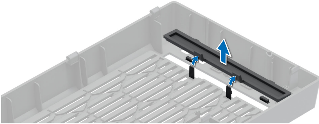
Ilustración 22. Extracción de las unidades ópticas de relleno del bisel frontal
