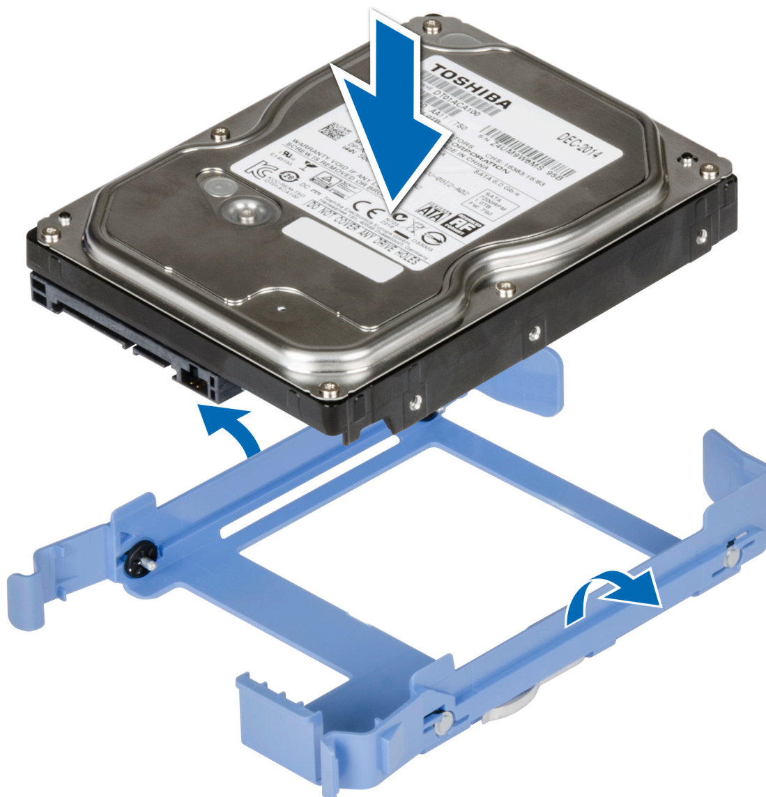
Ilustración 15. Instalación de una unidad en el portaunidades
