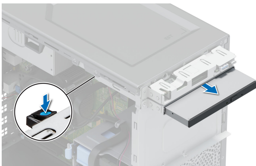
Ilustración 26. Extracción de las unidades ópticas
