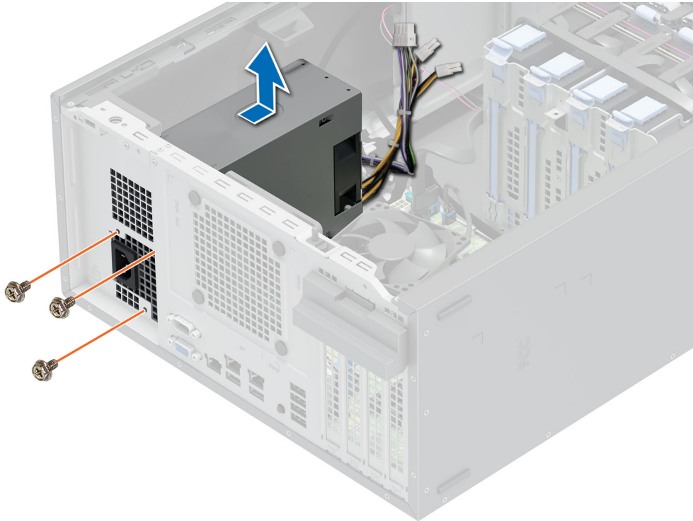
Ilustración 48. Extracción de la PSU D12
