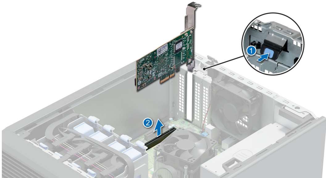
Ilustración 37. Extracción de la tarjeta de expansión PCIe
