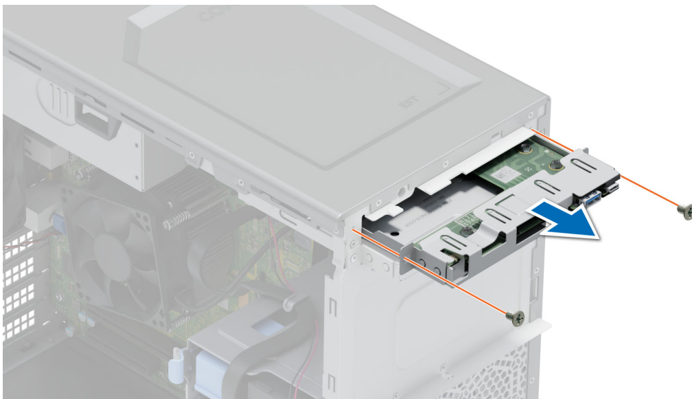
Ilustración 59. Extracción del compartimento del panel de control
