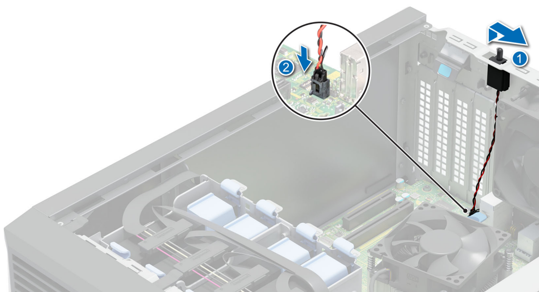
Ilustración 53. Instalación del interruptor de intrusiones
