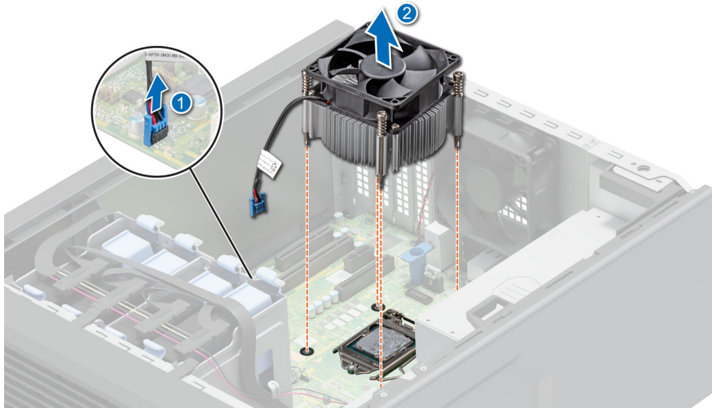
Ilustración 43. Extracción del disipador de calor
