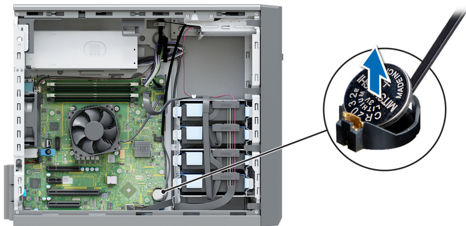
Ilustración 50. Extracción de la batería del sistema
