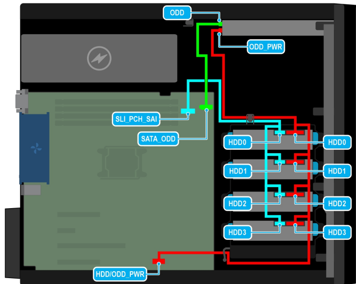
Ilustración 20. Enrutador de cables: unidad cableada de 4 x 3,5 pulgadas con SATA
