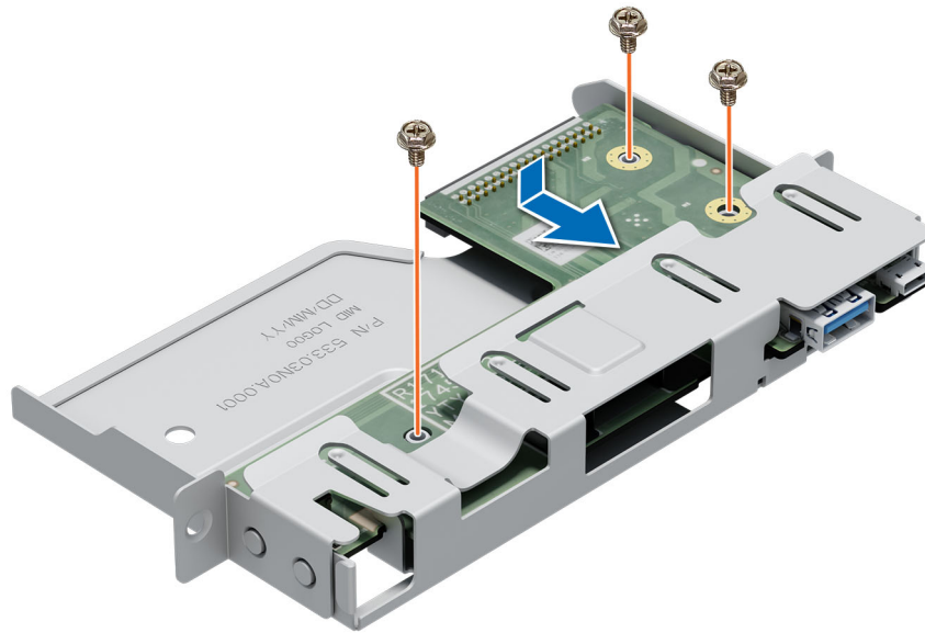
Ilustración 61. Instalación del panel de control
