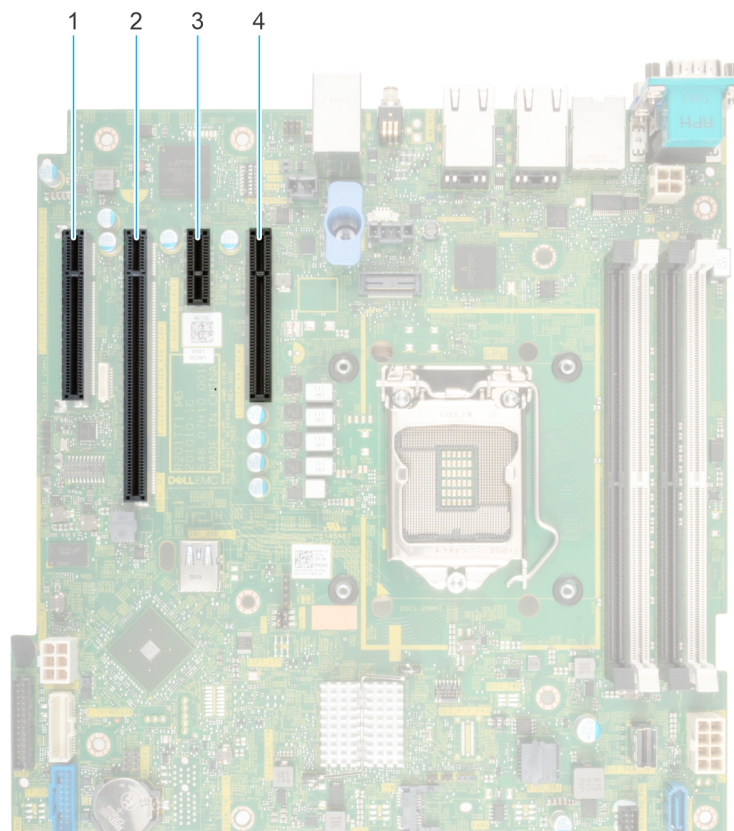
Ilustración 36. Conectores de la ranura de tarjetas de expansión
