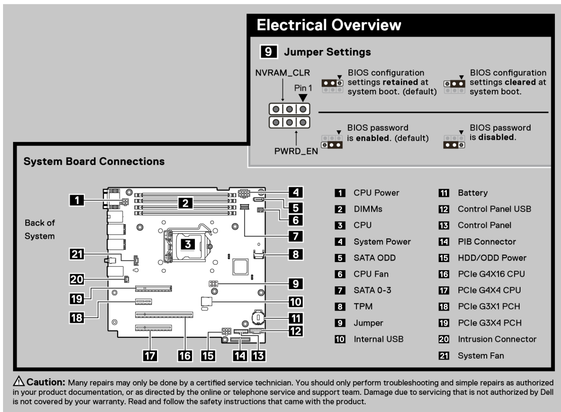
Ilustración 5. Características eléctricas generales y conexiones de la tarjeta madre
