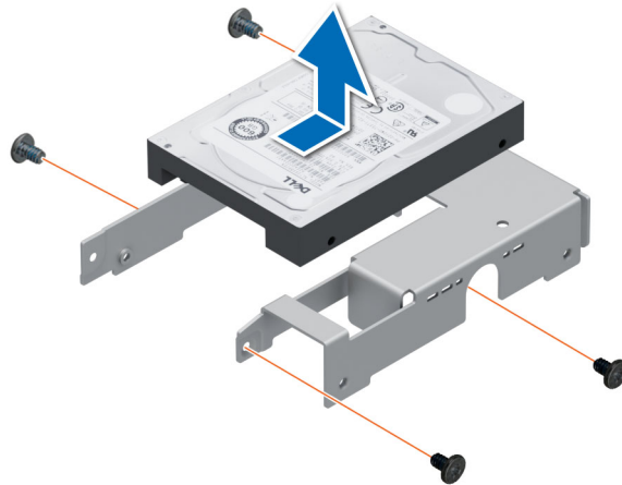
Ilustración 16. Extracción de una unidad de 2,5 pulgadas del adaptador de unidad de 3,5 pulgadas
