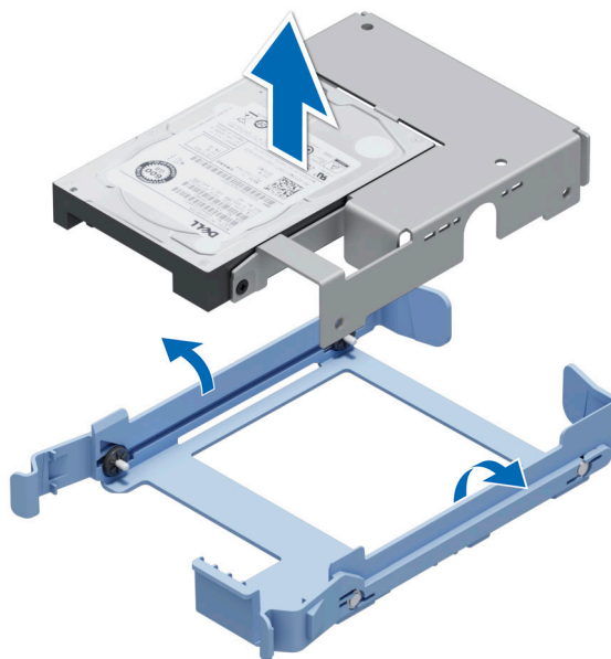
Ilustración 18. Extracción de un adaptador de unidad de 3.5 pulgadas de un portaunidades de 3.5 pulgadas
