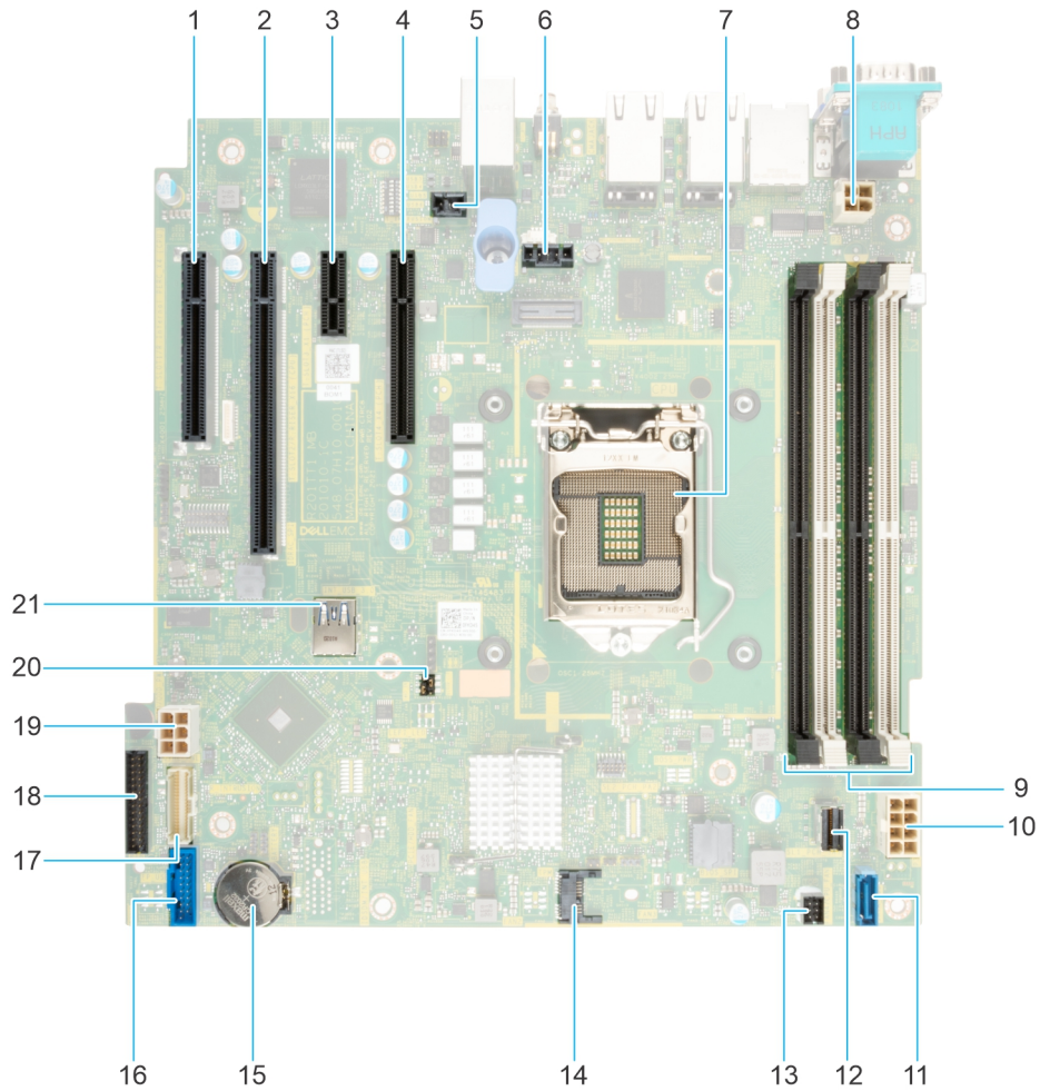
Ilustración 63. Puentes y conectores de la tarjeta madre del sistema
