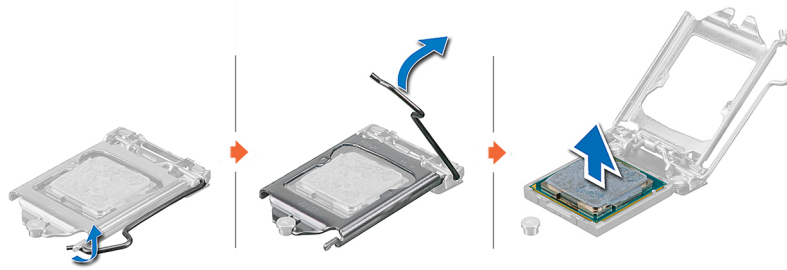
Ilustración 44. Extracción del procesador
