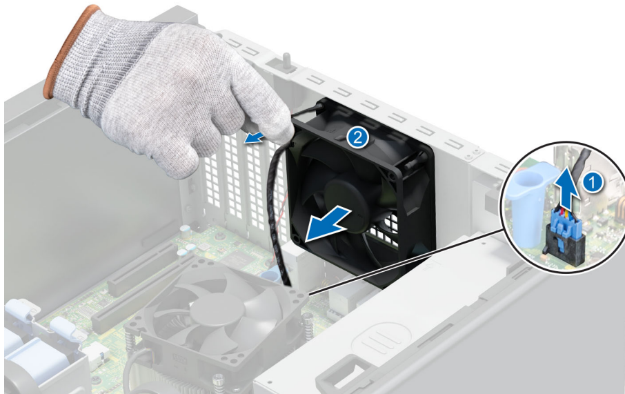
Ilustración 32. Extracción del ventilador de refrigeración
