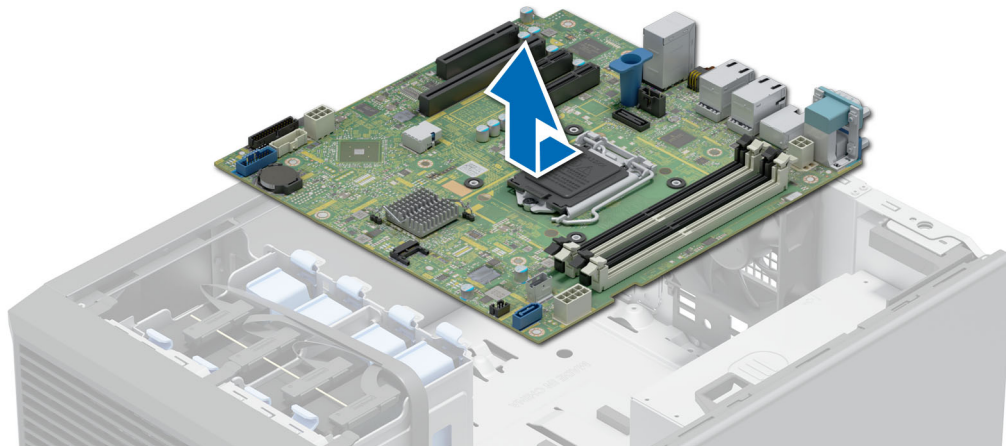
Ilustración 55. Extracción de la tarjeta madre
