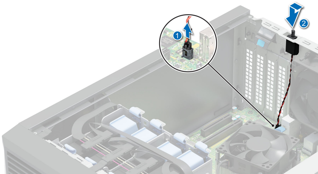
Ilustración 52. Extracción del interruptor de intrusiones
